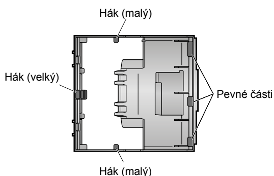
Zadní strana jednotky dezodorizačního filtru
